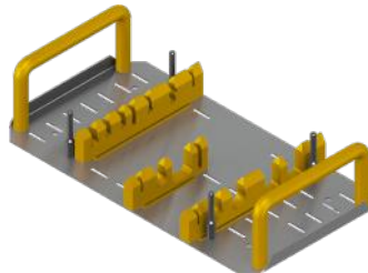
Conjunto Disposição de Instrumentais Sistema Cônico 5.0 Set of Instrumentation Conical System 5.0 Conjunto Disposición de Instrumentales Sistema Cônico 5.0 1.00.00.50.14.240
