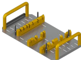
Conjunto Disposição de Instrumentais Sistema Cônico 7.0 Set of Instrumentation Conical System 7.0 Conjunto Disposición de Instrumentales Sistema Cônico 7.0 1.00.00.70.10.240
